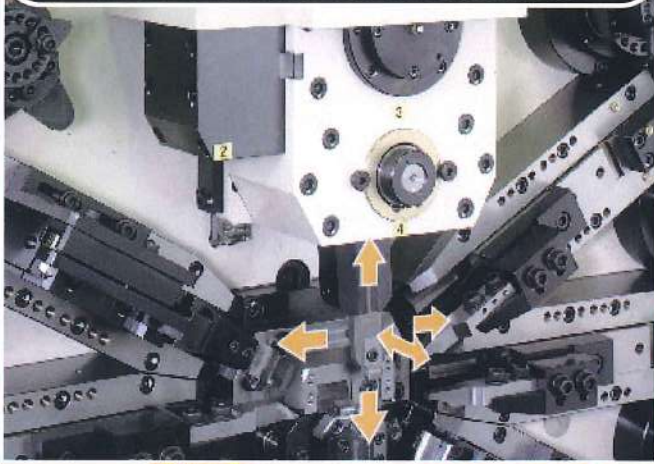
3次元トーションアタッチメント Three Dimensional Torsion Attachment
