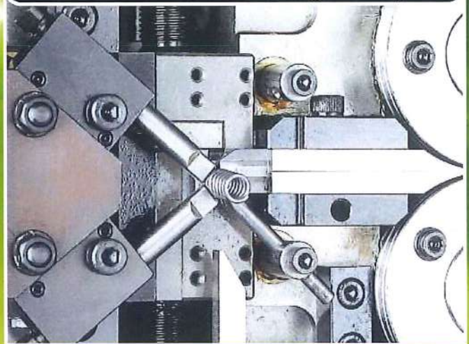
2本曲ユニット(オプション) / Two-finger Unit (Option)
