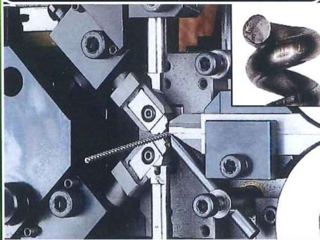
ハイパーカット(オプション) / Hyper Cutting Unit (Option)
