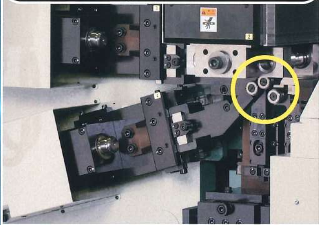
サーボコイリングにより曲率微小変化が可能 Servo Coiling for Variable Diameter
