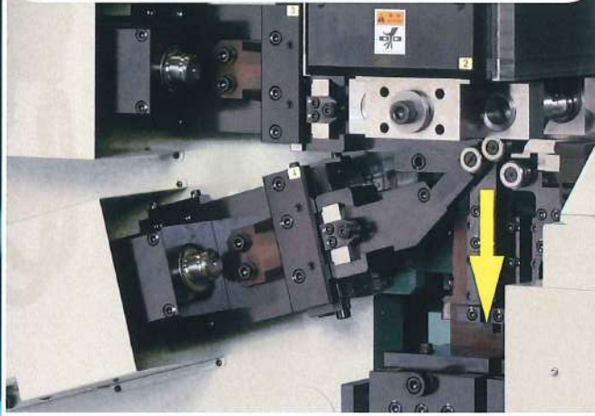
縦巻自由落下方式による高速度生産 High Speed Production
