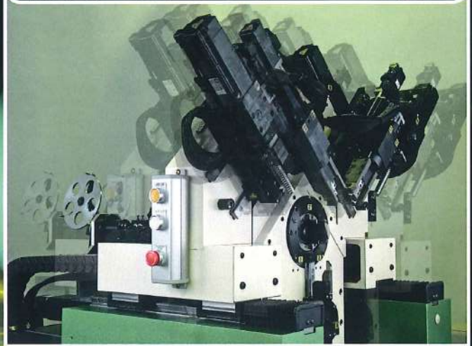
3次元移動ユニット / Three-Dimensional Moving Units
