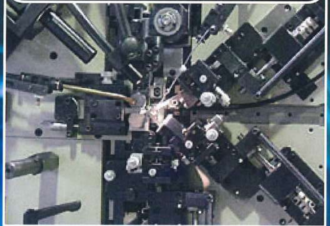
マイクロメーターによる曲ダイスの位置調整 Coiling Point Adjustment with Micrometers
